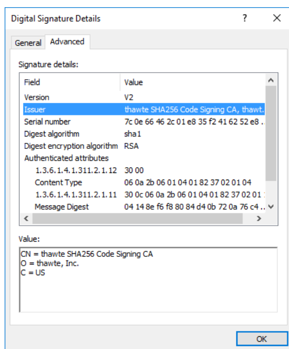
Slika 5: Prikaz digitalnega potrdila s katerim je podpisan namestitveni program
